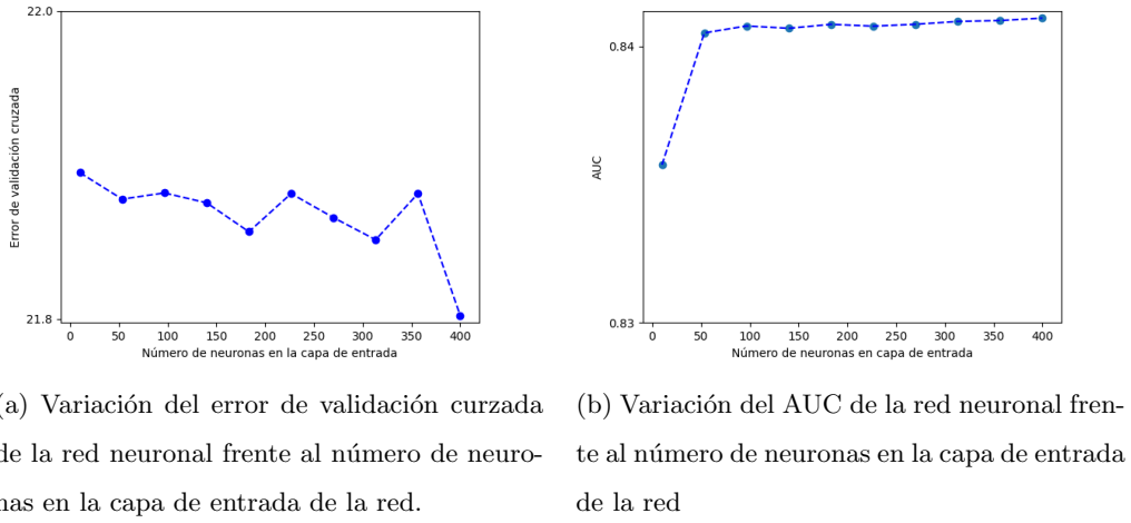
Figura 6.6: Variación del rendimiento de la red neuronal en función del número de neuronas en la capa de entrada.
