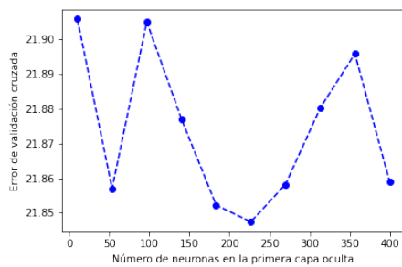
(a) Variación del error de validación cruzada de la red neuronal frente al número de neuronas en la primera capa oculta de la red.
