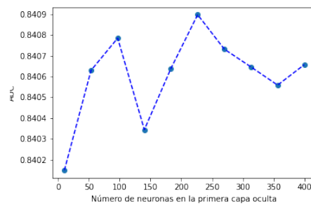
(b) Variación del AUC de la red neuronal frente al número de neuronas en la primera capa oculta de la red
