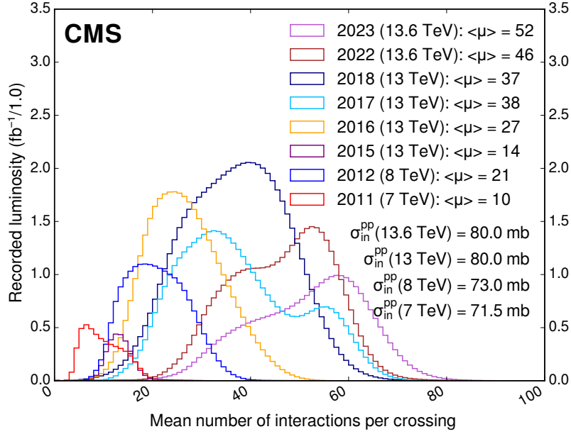
Figura 2.2: Representación gráfica del aumento del número de interacciones de pile up por colisión principal en el LHC, a lo largo de los años, debido al aumento de la luminosidad instantánea y la sección eficaz. [9]
