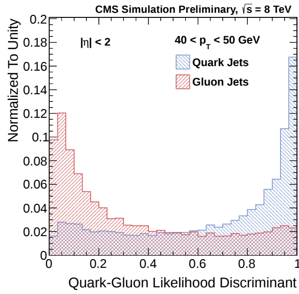
Figura 3.8: Representación gráfica de la distribución del discriminador de probabilidad, para jets originados por quarks ligeros y por gluones, para eventos dijet simulados con 40 < p_t < 50 \text{ GeV} y |\eta| < 2 . Se observa que alcanza un máximo cercano a 1 para los jets originados por quarks ligeros, mientras que el valor máximo para los jets generados por gluones es cercano a 0. [25]
