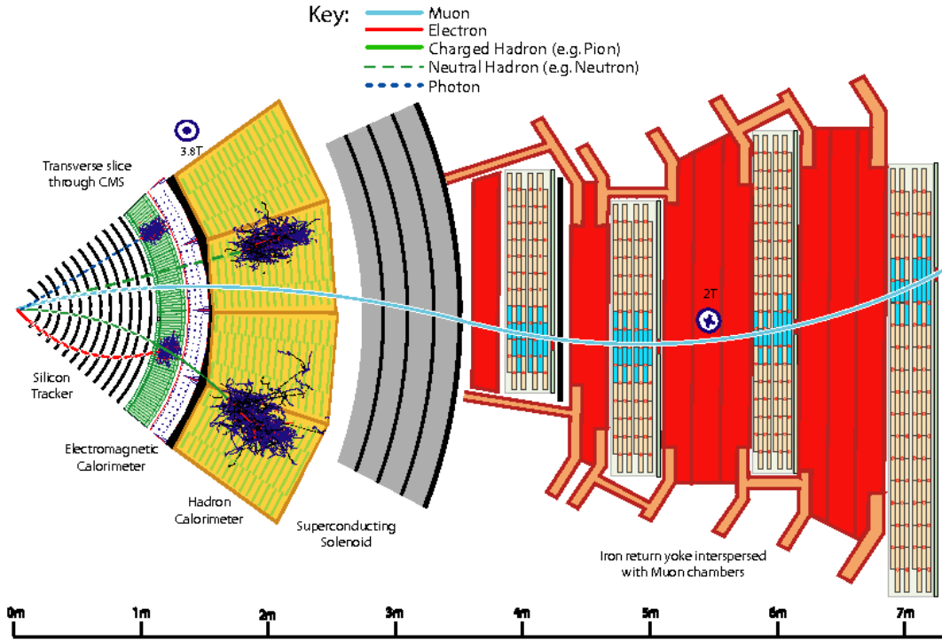
Figura 2.6: Esquema del recorrido de los diferentes tipos de partículas a través de CMS. Se observa como los electrones y fotones pierden toda su energía en el ECAL, y no avanzan más por el detector, mientras que los hadrones serán frenados en el calorímetro de hadrones. Por otro lado, los muones atraviesan todo el detector, hasta los detectores de muones. [16]
