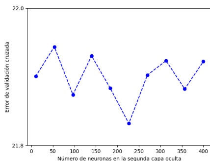
(a) Variación del error de validación cruzada de la red neuronal frente al número de neuronas en la segunda capa oculta de la red.
