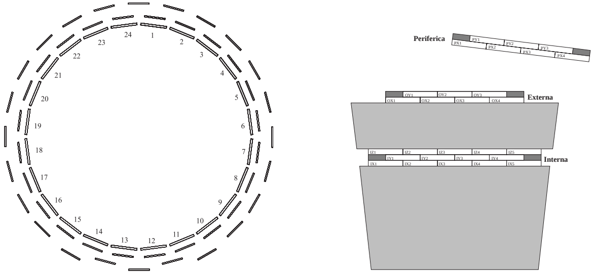
Figura 2.14: Vista frontal del MUB (izquierda) y colocación de módulos y cámaras (derecha).
