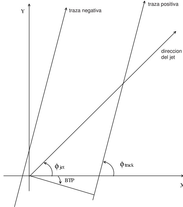
Figura 4.2: Esquema para el cálculo del signo del parámetro de impacto en el plano r\varphi
