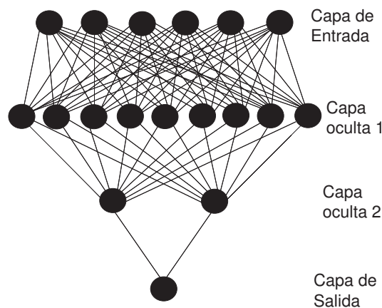
Figura 5.1: Ejemplo de arquitectura de un perceptrón multicapa:6-9-2-1.
