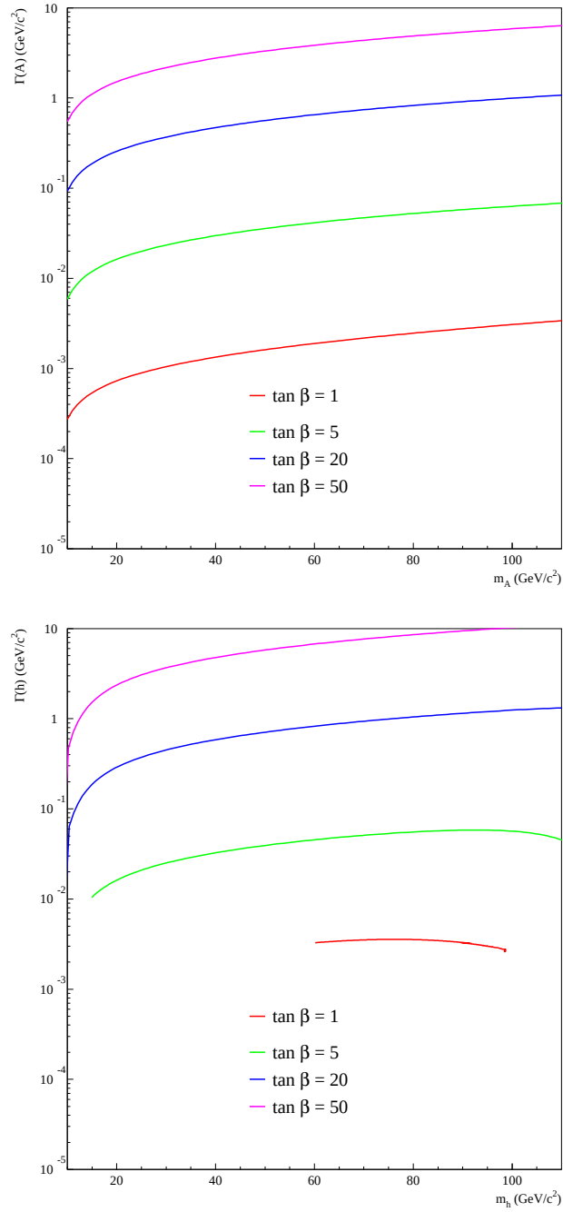
Figura 1.19: Anchuras totales de desintegración de los bosones A y h en función del parámetro \tan \beta . Para el caso del bosón h cuando \tan \beta = 1 , sus valores permitidos en el escenario m_h^{max} van desde 60 a \sim 90 \text{ GeV}/c^2 como se mostró en la figuras 1.13 y 1.14.
