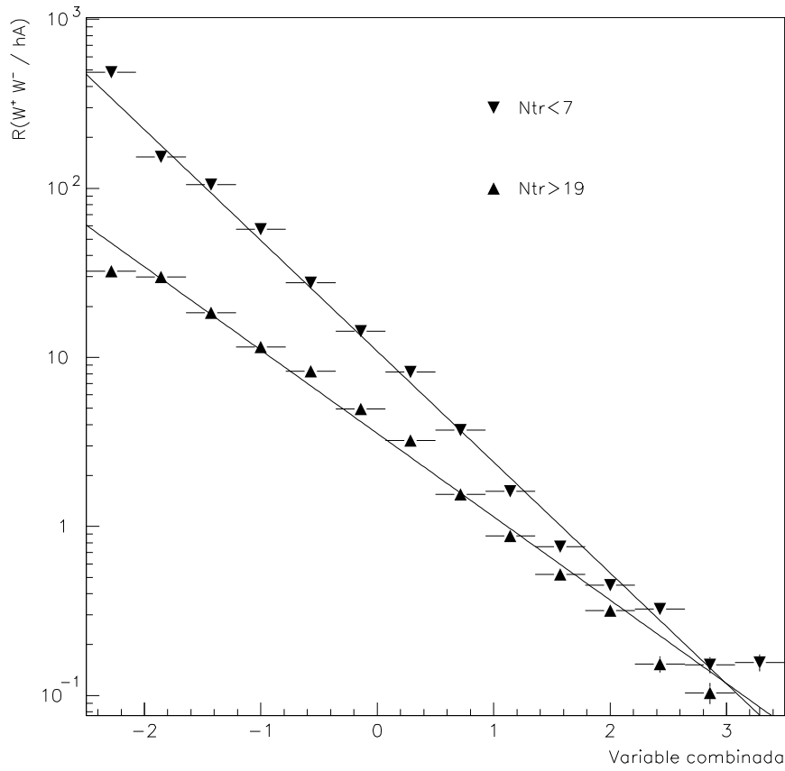
Figura 4.15: Distribución del cociente R(W^+ W^- / h^0 A^0) en función del valor de la variable combinada de b -tagging para jets con menos de 7 y más de 20 trazas cargadas. Las rectas son ajustes exponenciales a estos cocientes.
