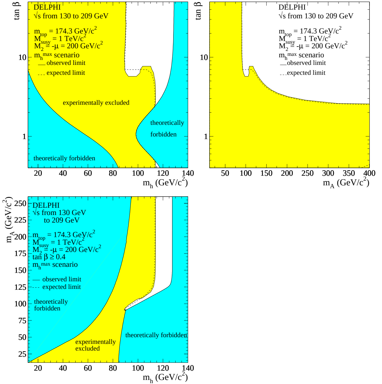
Figura 6.14: Regiones de exclusión al 95% de nivel de confianza por las búsquedas combinadas de los canales h^0 Z^0 y h^0 A^0 en el escenario m_h^{\max} . Las zonas en azul son regiones no permitidas en este escenario. Las líneas discontinuas muestran los límites esperados medios.
