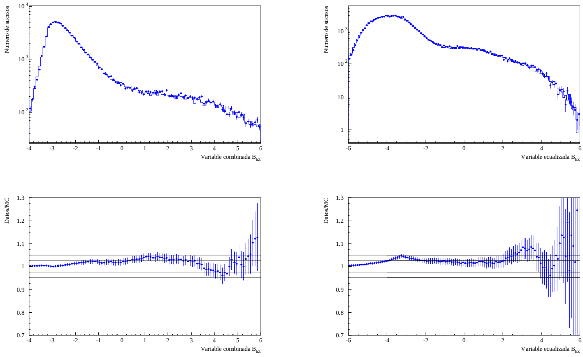
Figura 4.14: Acuerdo entre datos y simulación para la variable de suceso B_{hZ} usando sucesos hadrónicos Z^0 y b -tagging combinado (izquierda) y ecualizado h^0 Z^0 (derecha) en escala logarítmica (arriba) y el cociente datos/MC (abajo). Las discrepancias entre datos y simulación son inferiores al 5% tras introducir el proceso (segundo orden) de ecualización
