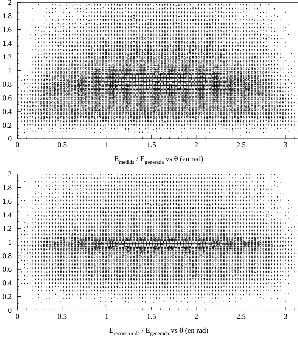
Figura 3.15: Distribución del cociente E/E_{\text{generada}} frente al ángulo \theta para la energía medida (superior) y la reconstruida (inferior) para sucesos simulados h^0A^0 con m_A = 90 \text{ GeV}/c^2 , \tan \beta = 20 .
