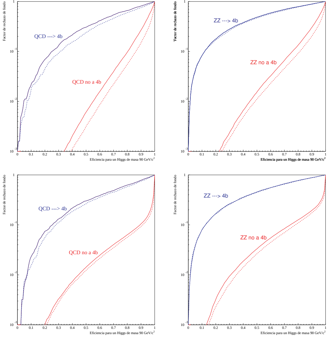
Figura 4.22: Comparación del rechazo de fondo en términos de contenido en quarks b para la variable B_{3+4} (arriba) y la variable B_{hA} (abajo) usando b -tagging combinado (línea continua) y b -tagging ecualizado h^0 A^0 (línea discontinua), para sucesos simulados de QCD (izquierda) y ZZ (derecha) y distinguiendo entre estados finales con 4 quarks b (azul) y el resto (rojo).
