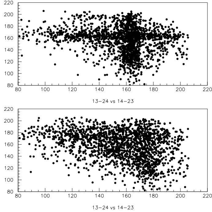
Figura 5.9: Suma de la masa de los dijets en la combinación 13-24 frente a la combinación 14-23 para sucesos h^0 A^0 con m_A = 90 \text{ GeV}/c^2 , \tan\beta = 2 (arriba) y \tan\beta = 50 (abajo), a \sqrt{s}=206.5 \text{ GeV} .
