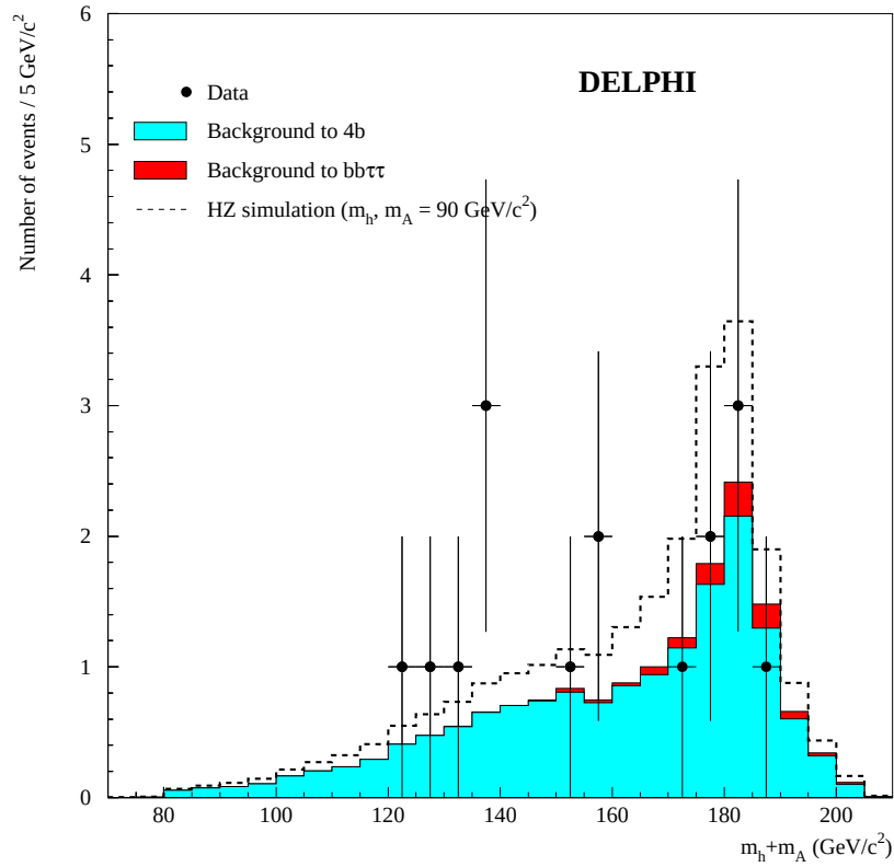
Figura 6.8: Distribución de masa combinada para el canal h^0 A^0 en DELPHI; esta figura es equivalente a la distribución del centro de la figura 5.10 salvo el fondo del canal bb\tau^+\tau^- (en rojo) que no presenta ningún candidato en datos.
