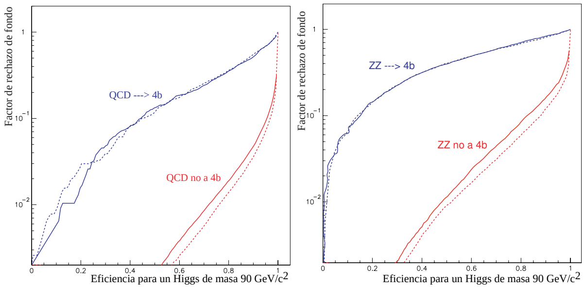
Figura 5.14: Comparación de rechazo de fondo frente a la eficiencia de una señal h^0 A^0 de masa 90 GeV/c 2 cortando en la variable RN (línea discontinua) y en la variable de tipo Likelihood (línea continua) del análisis previo de DELPHI para el fondo QCD (arriba) y el ZZ (abajo) distinguiendo entre los estados finales que tienen cuatro quarks de tipo b (en azul) y los que no (en rojo).
