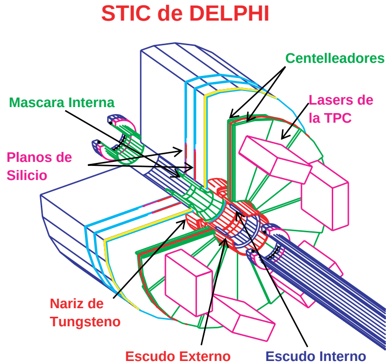
Figura 2.16: Disposición de los distintos componentes del STIC.
