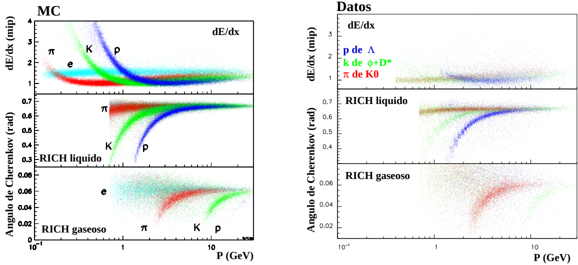
Figura 2.12: Valores de dE/dx en la TPC y del ángulo medio de Cherenkov en el RICH en función del momento para datos (derecha) y MC (izquierda).
