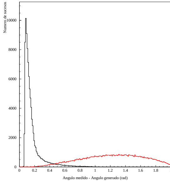
Figura 3.12: Diferencia angular en el espacio entre el jet generado y los 2 jets medidos más próximos (1° en negro y 2° en rojo) para sucesos h^0A^0 simulados con masa 90 GeV/ c^2 .
