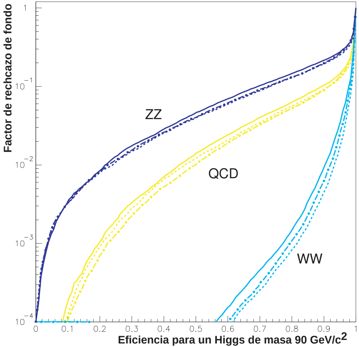
Figura 4.21: Rechazo de fondo frente a la eficiencia de la señal h^0 A^0 cortando en la variable de suceso B_{hA} usando: b -tagging combinado (línea continua), b -tagging ecualizado (línea discontinua) y b -tagging ecualizado usando la señal h^0 Z^0 (línea a trazos y puntos).
