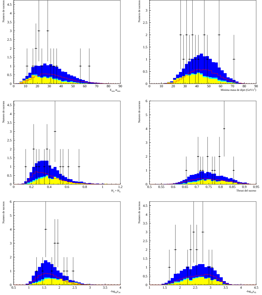
Figura 5.12: Distribuciones de las 6 primeras variables de entrada de la RN a S/B \simeq 1.0 . De arriba a abajo y de izquierda a derecha: E_{\min} \alpha_{\min} , minima masa de dijet, H_2 + H_4 , thrust del suceso, -\log_{10}(y_{34}) y -\log_{10}(y_{45})
