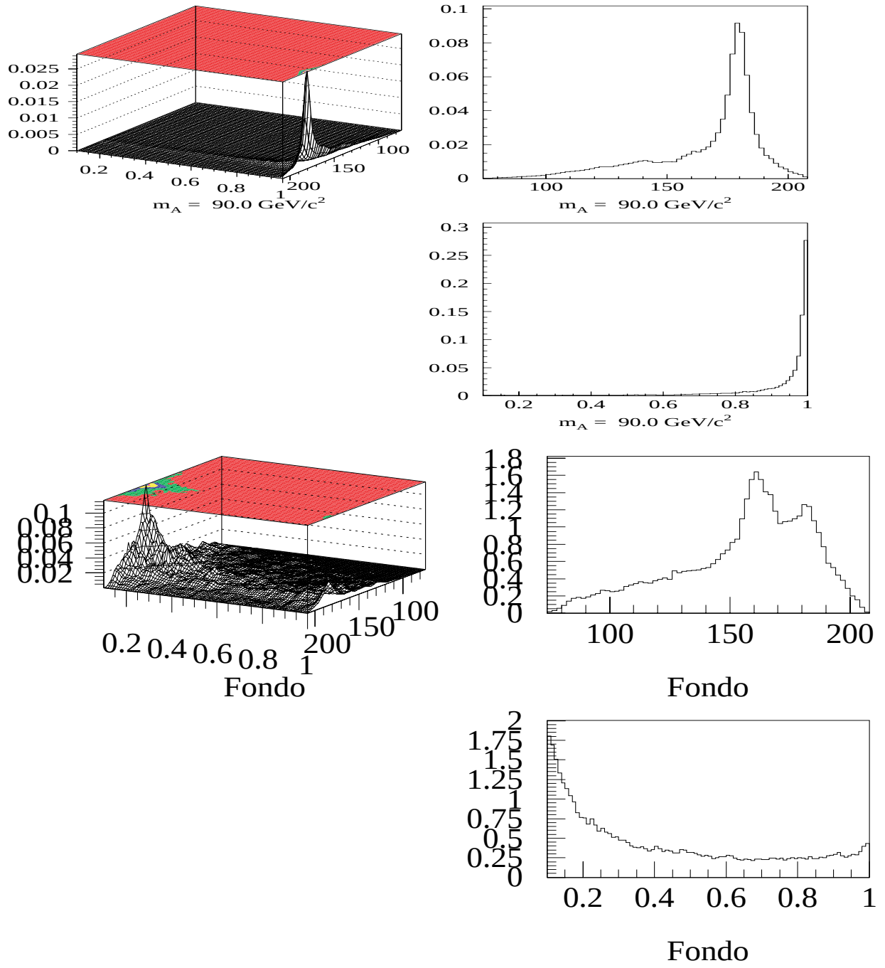
Figura 6.3: Distribuciones bidimensionales ( m_A, R_N ) y sus proyecciones para una señal m_A=90 \text{ GeV}/c^2 (arriba) y el fondo del canal 4b (abajo) a \sqrt{s}=206.5 \text{ GeV} .
