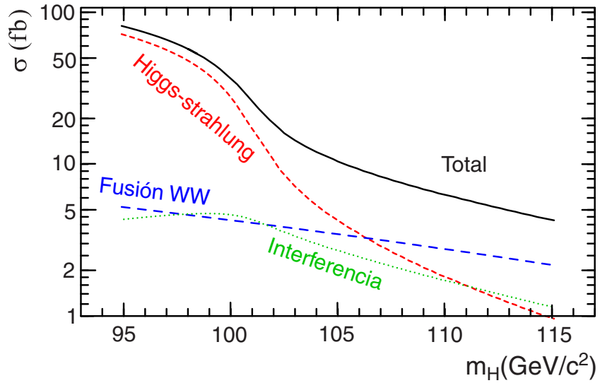
Figura 1.4: Comparaci3n entre las secciones eficaces de los procesos de Higgs-strahlung y fusi3n W^+W^- en funci3n de la masa del bos3n de Higgs para el caso e^+e^- \rightarrow H\nu\bar{\nu} y \sqrt{s} = 192 GeV. La l3nea s3lida representa la secci3n eficaz total incluyendo los t3rminos de interferencia.
