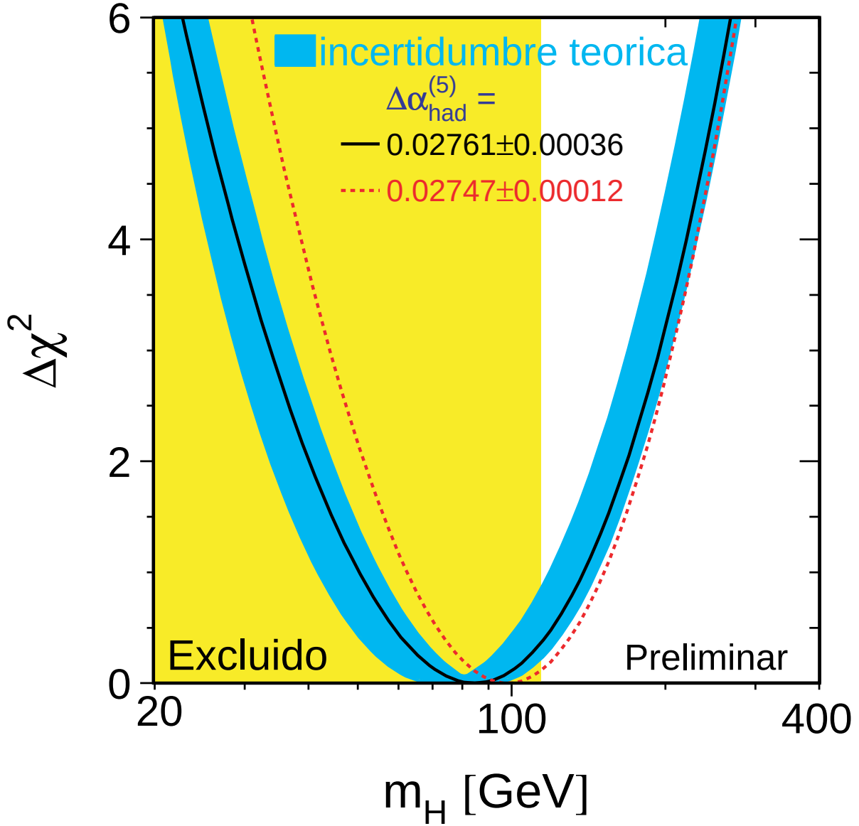
Figura 1.9: \Delta\chi^2 = \chi^2 - \chi_{\min}^2 en función de m_H calculado a partir de medidas de precisión electrodébiles. La banda sombreada es una estimación del error teórico debido a las correcciones de alto orden que no se están incluidas. La banda vertical muestra la región excluida para un 95% de nivel de confianza por búsqueda directa.
