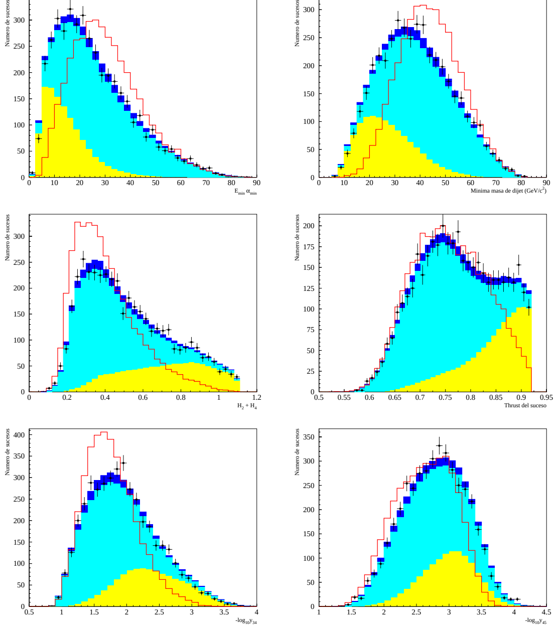
Figura 5.2: Distribuciones de las 6 primeras variables de entrada de la RN. De arriba a abajo y de izquierda a derecha: E_{\min} \alpha_{\min} , minima masa de dijet, H_2 + H_4 , thrust del suceso, -\log_{10}(y_{34}) y -\log_{10}(y_{45})
