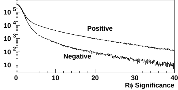
Figura 4.4: Valor absoluto de la significancia en r\phi para trazas con IP positivo (curva superior) y negativo (curva inferior) en sucesos hadrónicos Z^0 . El exceso de trazas con signo positivo con gran significancia es debido a partículas con larga vida media.
