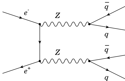
Figura 3.9: Diagrama de Feynman correspondiente al proceso e^+e^- \rightarrow ZZ .
