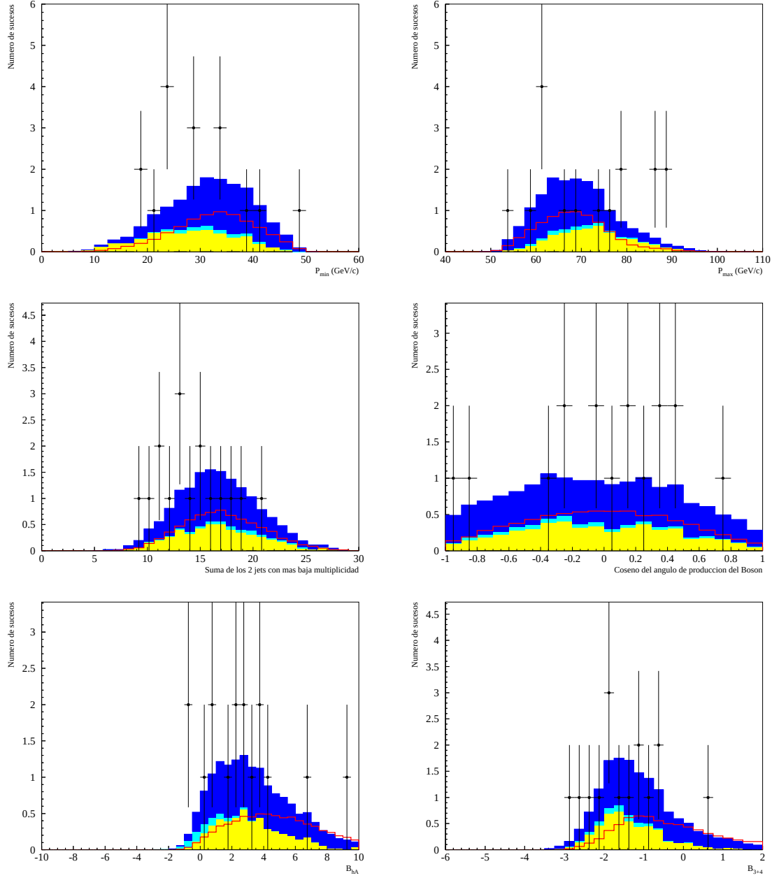
Figura 5.13: Distribuciones de las 6 restantes variables de entrada de la RN a S/B \approx 1.0 . De arriba a abajo y de izquierda a derecha: \vec{p}_{min} , \vec{p}_{max} , suma del número de trazas para los dos jets con menos trazas, coseno del ángulo de producción del Bosón, B_{hA} y B_{3+4}
