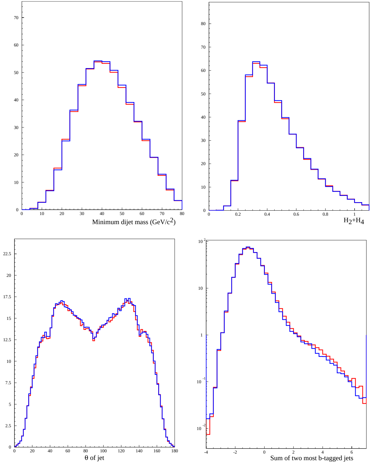
Figura A.2: Comparación del generador WPHACT (en rojo) frente a EXCALIBUR (en azul) en sucesos a 4f para cuatro variables: mínima masa de dijet (arriba izquierda), suma del segundo y cuarto momentos de Fox-Wolfram (arriba derecha), ángulo polar \theta del jet (abajo izquierda) y la variable de b -tagging para los dos jets más altos (abajo derecha).
