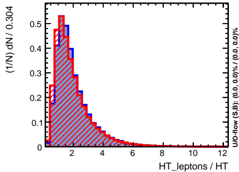
Input variable: HT_leptons / HT
